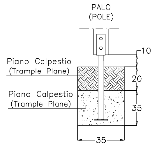
PARTICOLARI ANCORAGGIO (ANCHORAGE DETAIL)
