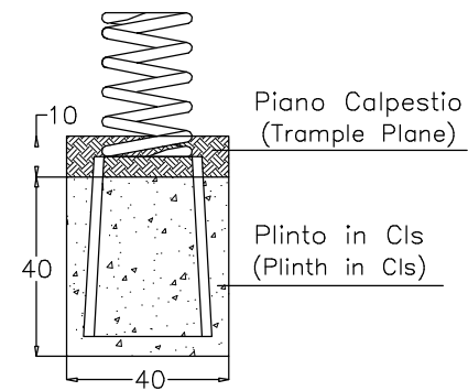
PARTICOLARI ANCORAGGIO (ANCHORAGE DETAIL)
