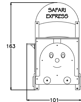
VISTA B LOCOMOTIVA
