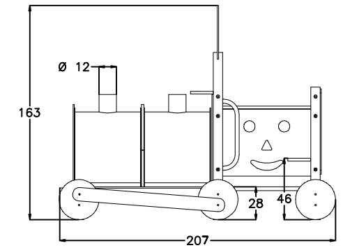
VISTA A LOCOMOTIVA
