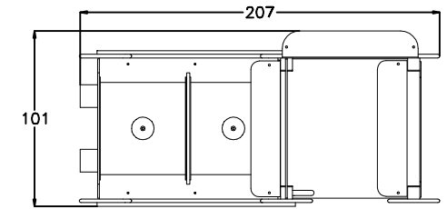
PIANTA LOCOMOTIVA
