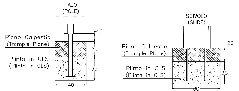
PARTICOLARI ANCORAGGIO (ANCHORAGE DETAIL)
