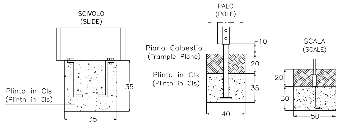
PARTICOLARI ANCORAGGIO (ANCHORAGE DETAIL)
