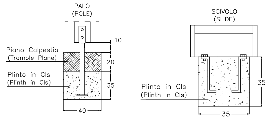
PARTICOLARI ANCORAGGIO (ANCHORAGE DETAIL)
