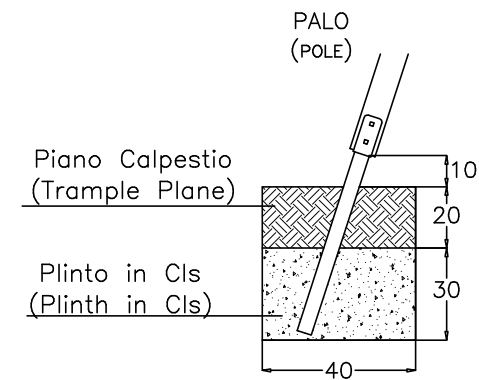
PARTICOLARI ANCORAGGIO (ANCHORAGE DETAIL)
