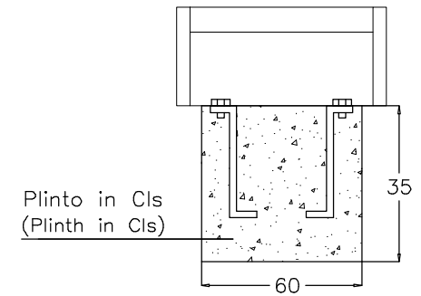
SCIVOLO (SLIDE)
