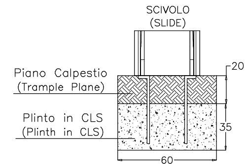
PARTICOLARI ANCORAGGIO (ANCHORAGE DETAIL)
