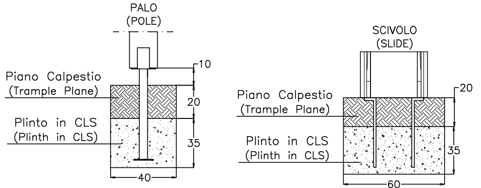
PARTICOLARI ANCORAGGIO (ANCHORAGE DETAIL)
