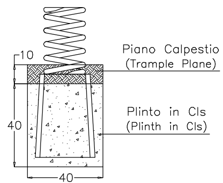
PARTICOLARI ANCORAGGIO (ANCHORAGE DETAIL)
